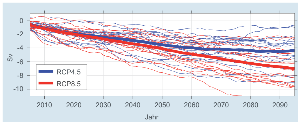
Abbildung 8: Die mit verschiedenen Klimamodellen für das 21. Jahrhundert projizierte und mit einem Zehn-Jahre-Filter geglättete Änderung der Umwälzzirkulation (Sv) bei 30^\circ \text{N} gegenüber 1970–2000, deren Ergebnisse im 5. Sachstandsbericht des Weltklimarats Eingang gefunden haben. Gezeigt sind Ergebnisse für zwei Treibhausgas-szenarien: Ein moderates Szenario (RCP4.5, blaue Linien) und ein „Worst-Case-Szenario“ (RCP8.5, rote Linien). Das RCP8.5 Szenario entspricht einer äquivalenten \text{CO}_2 -Konzentration von 1370 ppm (parts per million) gegen Ende des 21. Jahrhunderts gegenüber 650 ppm im RCP4.5 Szenario. Die Mittelwerte über alle Modelle sind als fette Linien gezeigt. Die Stärke der Umwälzzirkulation bei 26,5^\circ \text{N} im Zeitraum 1970–2000 beträgt im Mittel über alle Modelle 19 Sv. Die gemessene Stärke bei 26,5^\circ \text{N} lag von April 2004 bis Oktober 2015 bei 16,9 \pm 4,4 \text{ Sv} .
