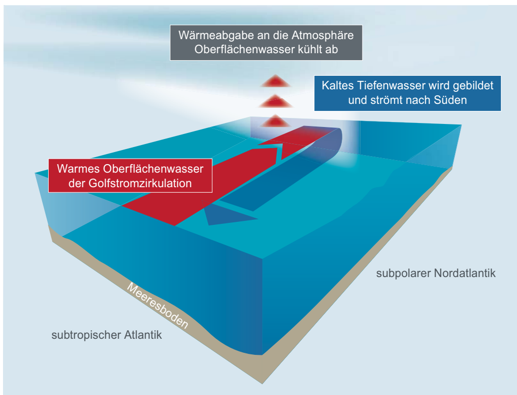
Abbildung 2: Schematische Darstellung der durch Temperaturänderungen und durch Salzgehaltsänderungen (daher „thermohalin“) angetriebenen Zirkulation, die als Umwälzzirkulation bezeichnet wird.
